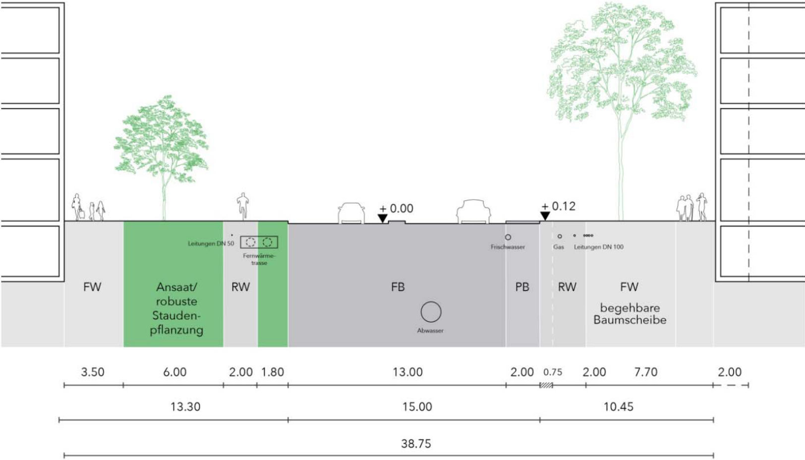
Abb. Straßenquerschnitt Römerstraße – Variante 1
