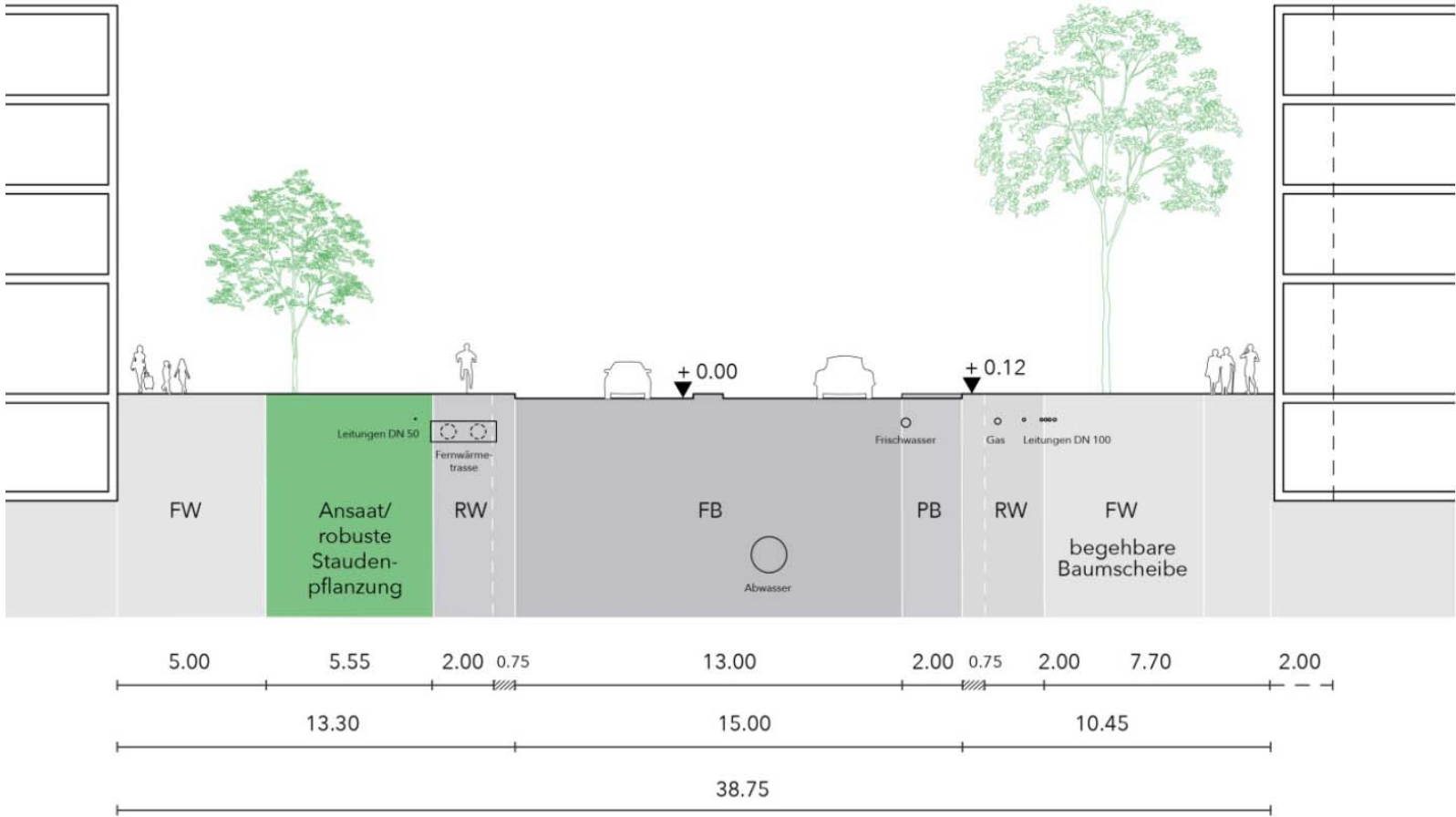
Abb. Straßenquerschnitt Römerstraße – Variante 2
