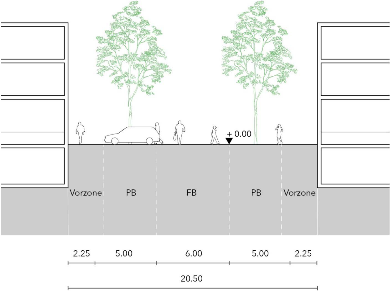
Abb. Wohnweg östlich Römerstraße
