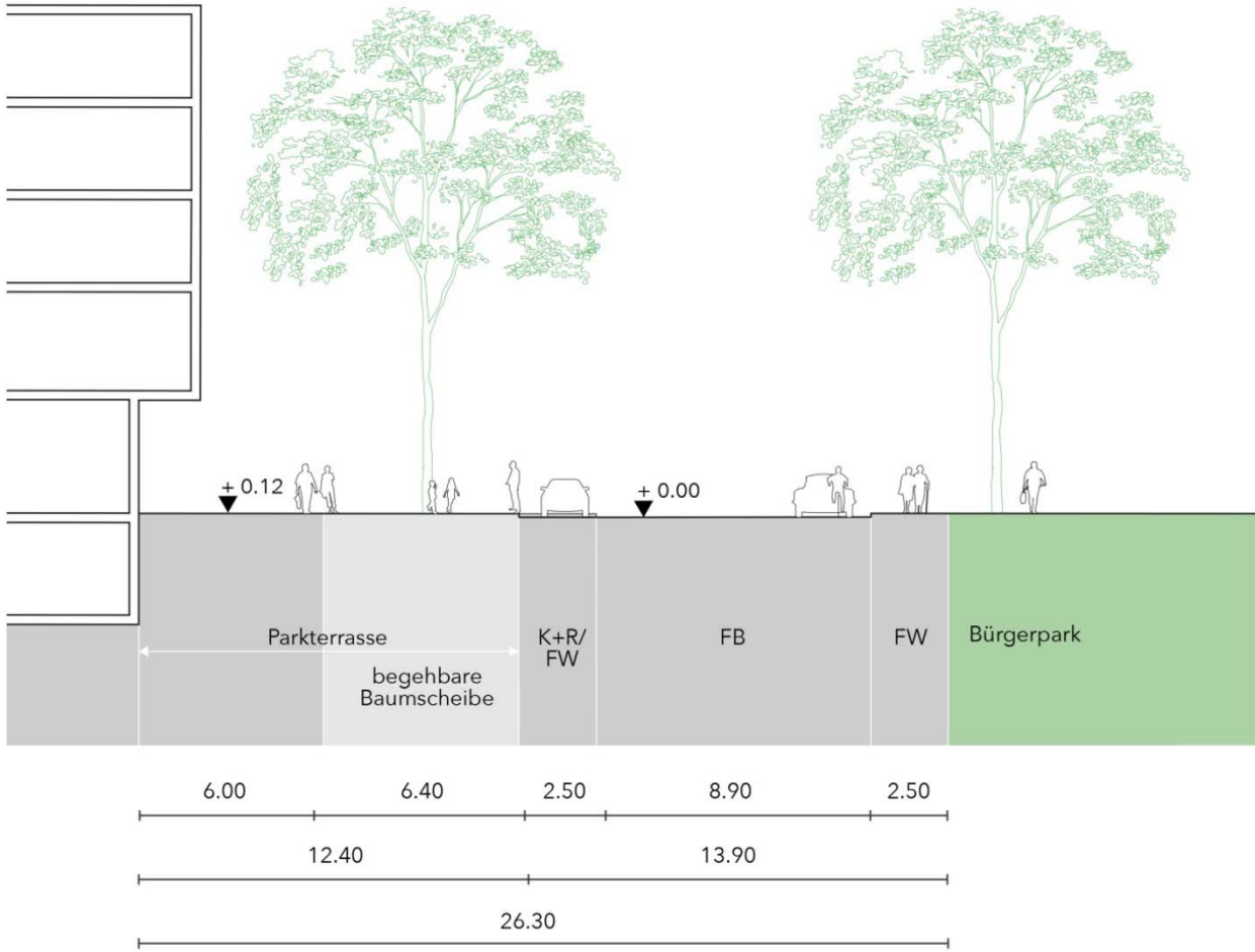
Abb. Straßenquerschnitt Rheinstraße
