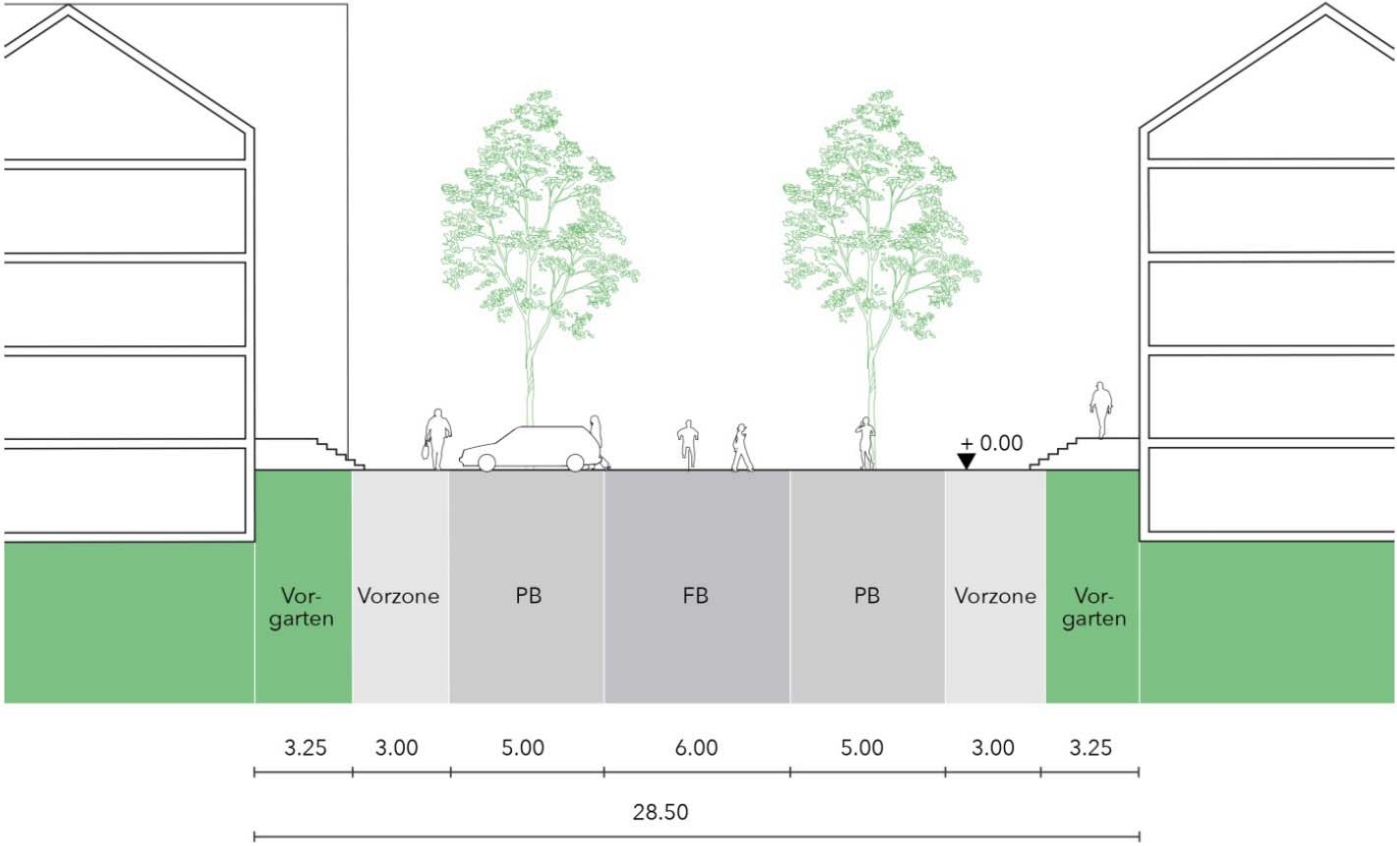
Abb. Wohnweg westlich Römerstraße
