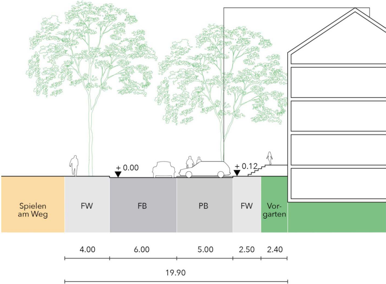
Abb. Straßenquerschnitt Elsa-Brandström-Straße
